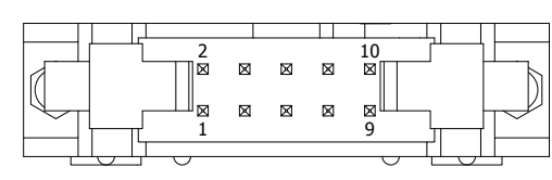
DETAIL A 3M# 3793-5303
